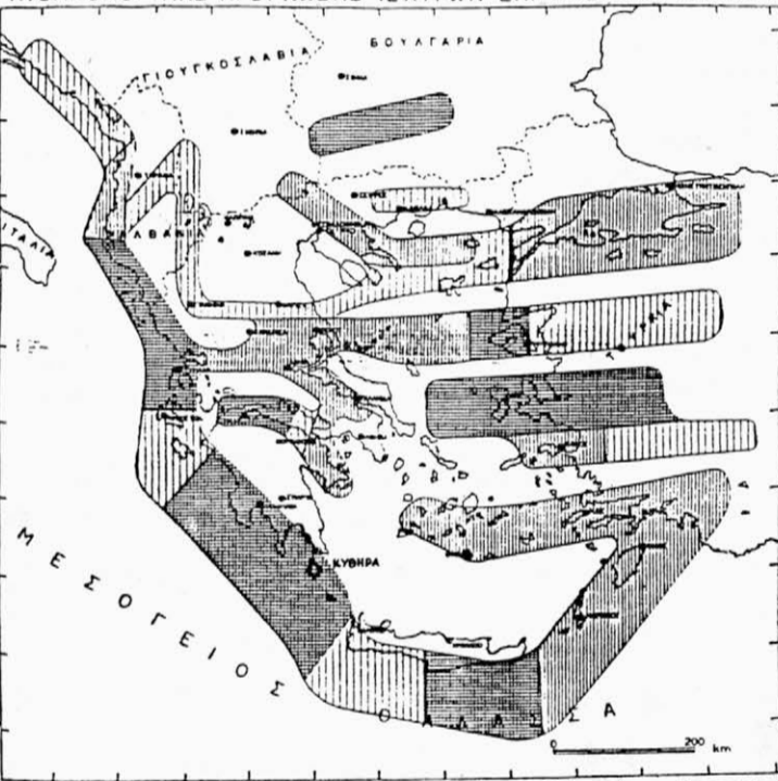
ΧΑΡΤΗΣ ΠΙΘΑΝΟΛΟΓΙΚΗΣ ΠΡΟΓΝΩΣΗΣ ΙΣΧΥΡΩΝ ΕΠΙΦΑΝΕΙΑΚΩΝ ΣΕΙΣΜΩΝ
