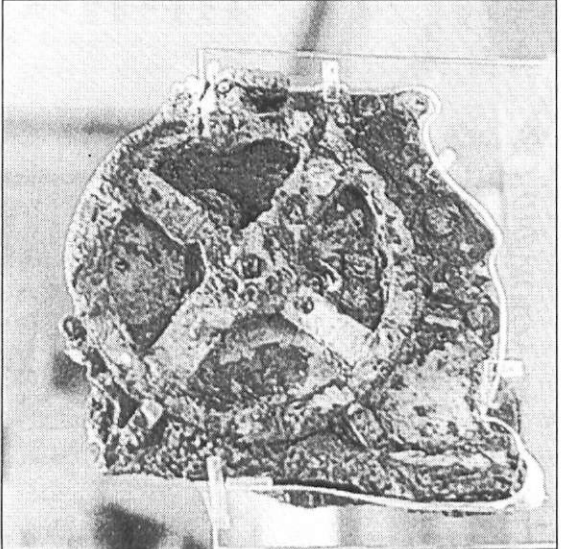
Ο Μηχανισμός των Αντικυθήρων ανελκύθη σε πολλά κομμάτια. Εδώ είναι το κυριότερο. Σε πρόσφατη έκθεση στο Πολεμικό Μουσείο, απ' όπου η φωτογραφία, απεκαλύφθη ότι ο μηχανισμός διέθετε 40 γρανάζια (αντί των 32 που πίστευαν μέχρι τώρα οι ειδικοί) τα οποία εκκινούν συγχρονισμένα. Ένα επίτευγμα τεχνολογίας δύο χιλιάδων χρόνων!
