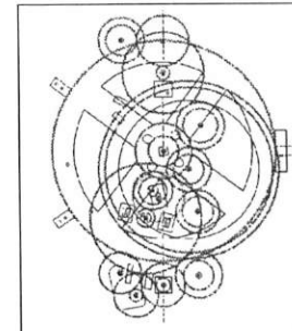
Απόπειρες σχεδιασμού του κύριου τμήματος του Μηχανισμού.
